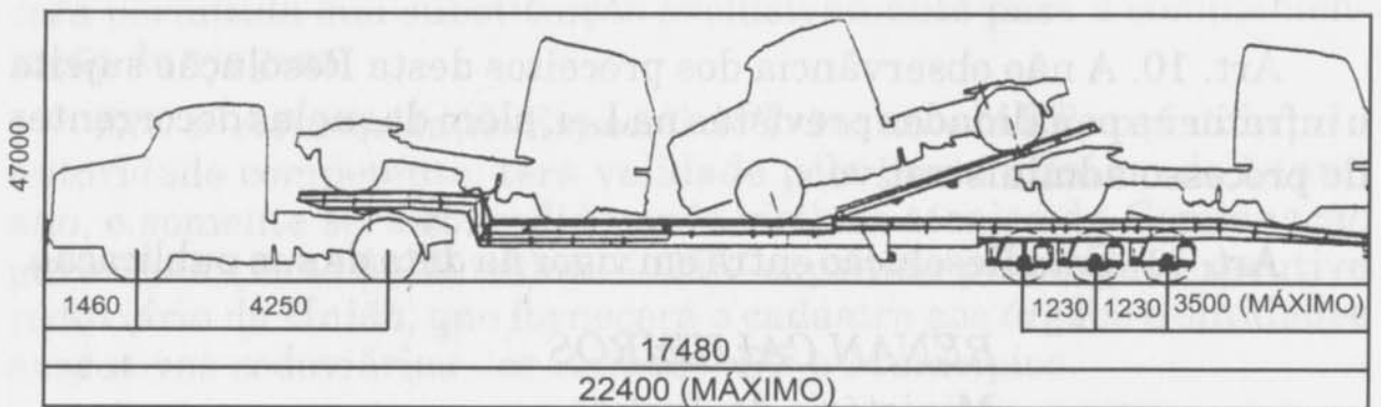
Semi-Reboque Transporte Caminhões e Ônibus
