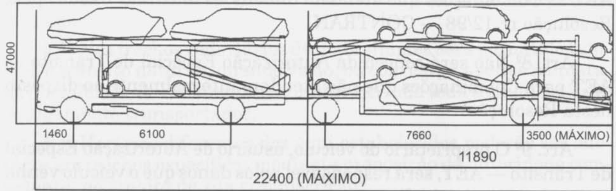
Cavalo Trator e Reboque
