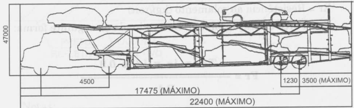
Semi-Reboque Transporte Automóveis
