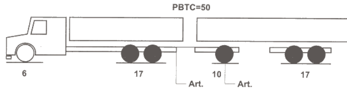
Romeu e Julieta comprimento 19,80 m Duas Articulações
