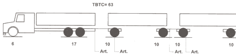
Treminhão comprimento 30,00 m Quatro articulações
