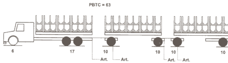
Treminhão comprimento 30,00 m Quatro Articulações
