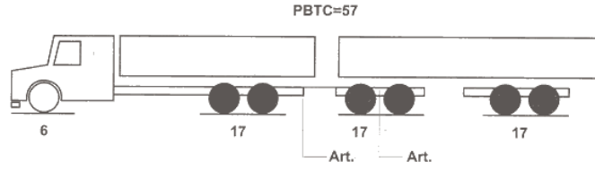
Romeu e Julieta comprimento 19,80m Duas Articulações
