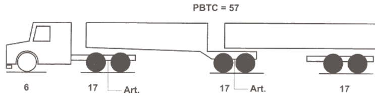
Bi Trem Articulado comprimento 19,80 m Duas Articulações
